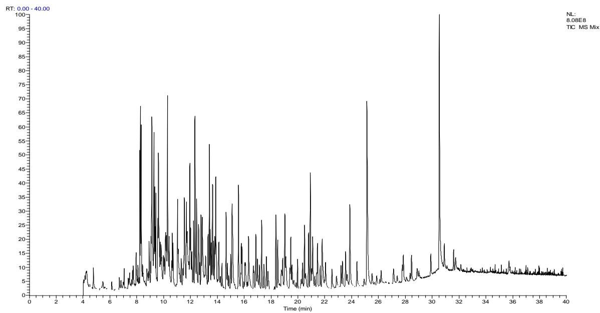
图B. 1 空白血液中添加 188 种毒(药)物和内标的色谱图
